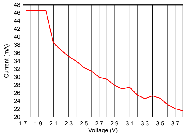
图 7-13. TX 电流与电源电压 (VDD) 间的关系 ( BLE 1Mbps , 2.44GHz , +10dBm )
