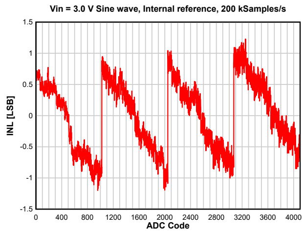
图 8-32. INL vs. ADC Code
