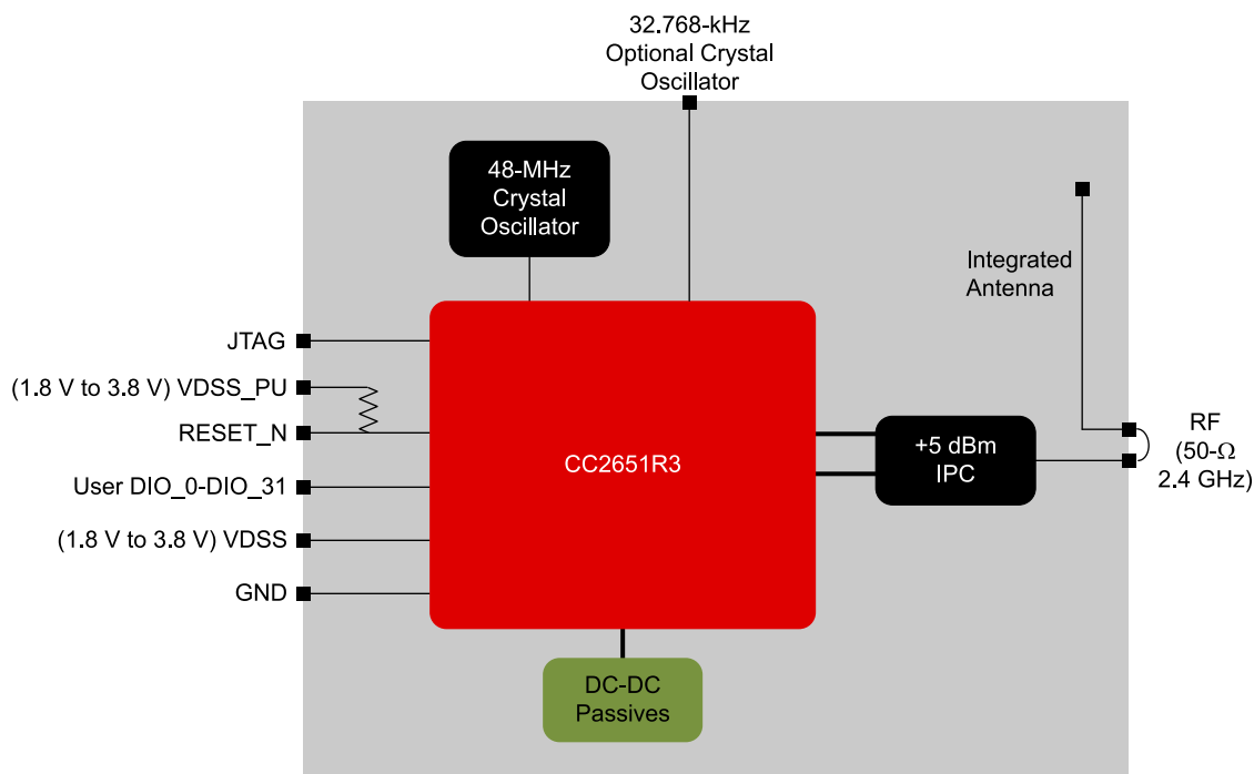
图 4-1. CC2651R3SIPA 方框图
