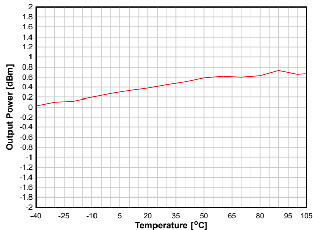
图 8-16. Output Power vs. Temperature(BLE 1 Mbps, 2.44 GHz, 0dBm)
