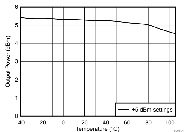
图 7-7. TX Output Power vs Temperature
