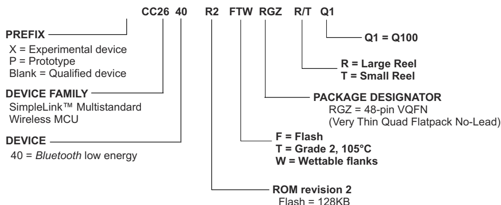
图 10-1. Device Nomenclature
