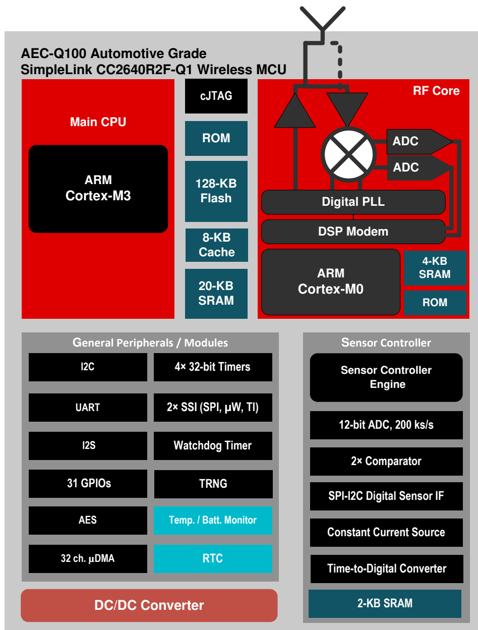
方框图
