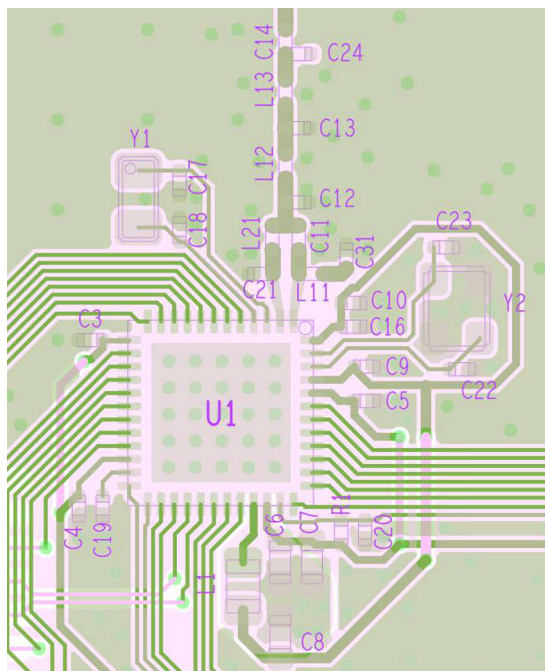
图 9-4. Layout
