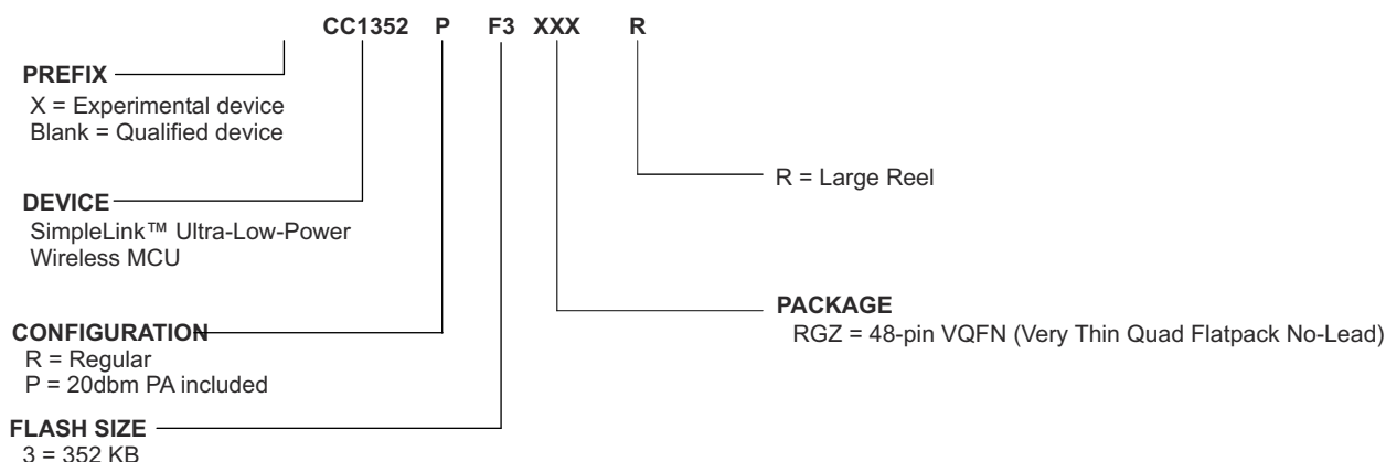
图 11-1. Device Nomenclature
