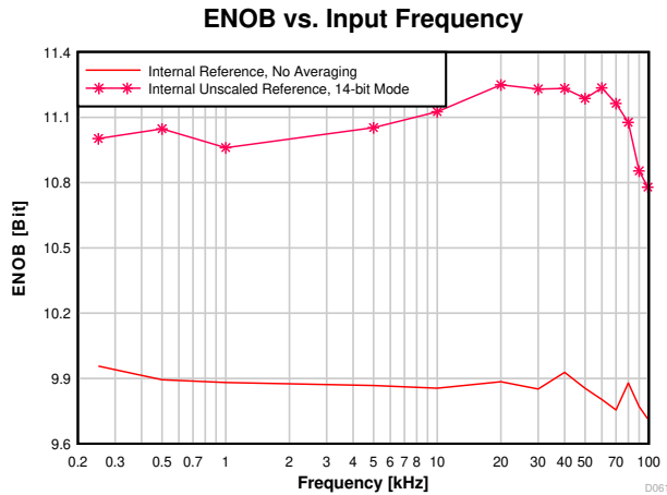
图 8-25. ENOB 与输入频率间的关系
