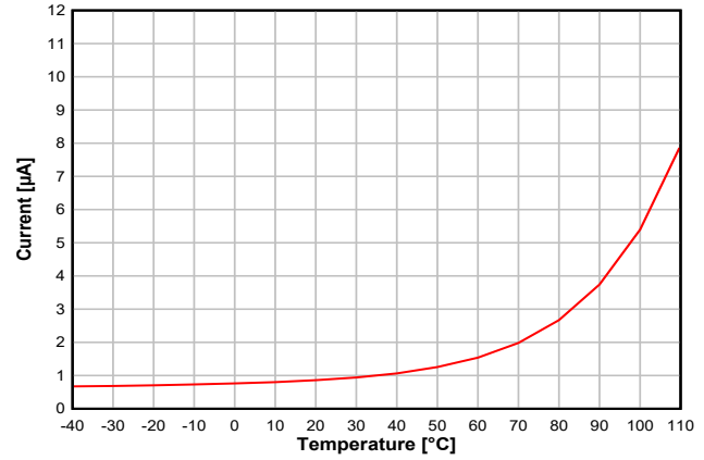
图 8-5. 待机模式 (MCU) 电流与温度间的关系 (80kB RAM 保留, 无高速缓存保留, RTC On SCLK_LF = 32kHz XOSC)
