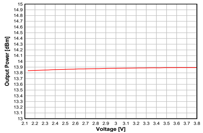
图 8-22. 输出功率与电源电压 (VDD5) 间的关系 ( 915MHz , +14dBm 设置 )
