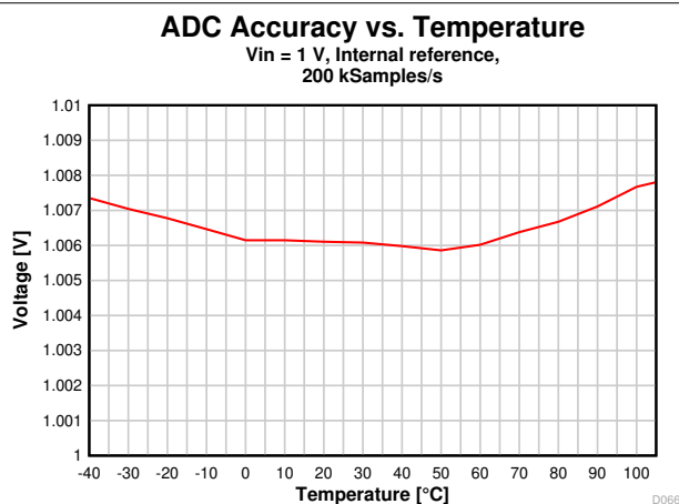
图 8-29. ADC 精度与温度间的关系
