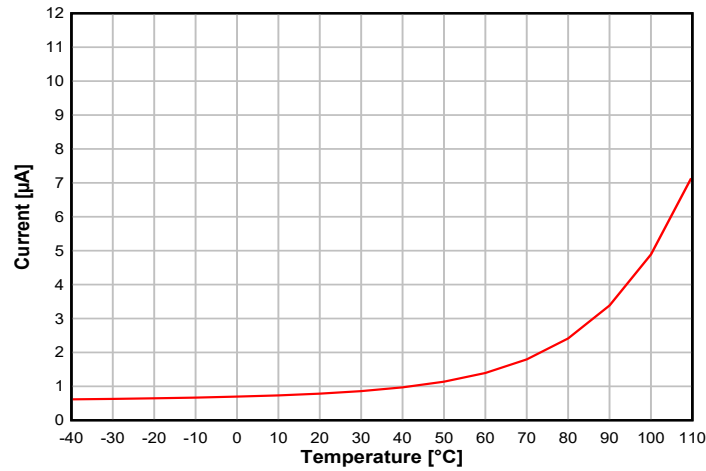
图 8-6. 待机模式 (MCU) 电流与温度间的关系 (80kB RAM 保留, 无高速缓存保留, RTC On SCLK_LF = 32kHz XOSC, VDD5 = 3.6V)
