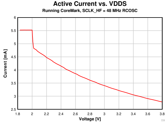
图 8-4. 工作模式 (MCU) 电流与电源电压 (VDD5) 间的关系 (运行 CoreMark 时, SCLK_HF = 48MHz RCOSC)
