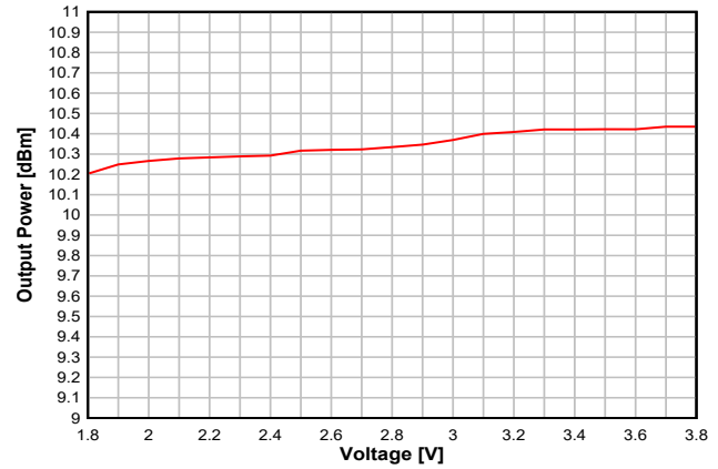
图 8-20. 输出功率与电源电压 (VDD5) 间的关系 ( 868.3MHz , +10dBm 设置 )
