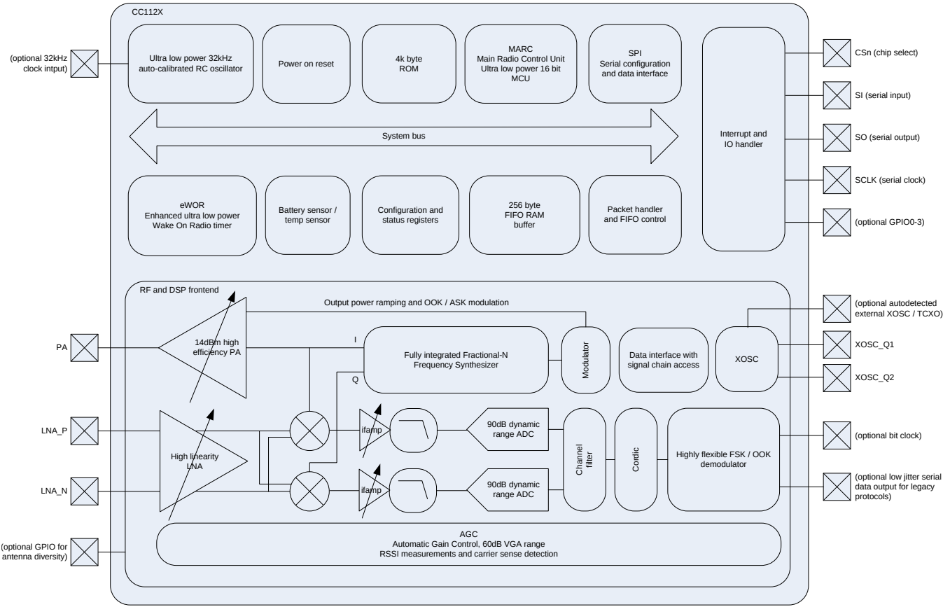
图 1-1. 功能方框图
