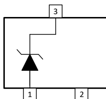
图 5-1. DCK 封装, 3 引脚 SC-70 (顶视图)
