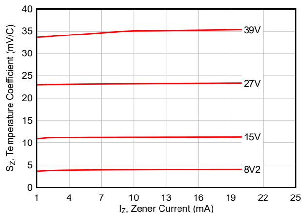
图 6-2. 温度系数
