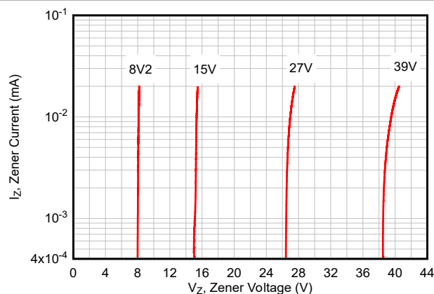
图 6-1. 齐纳电流与齐纳电压间的关系
