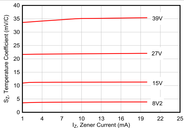
图 5-2. 温度系数
