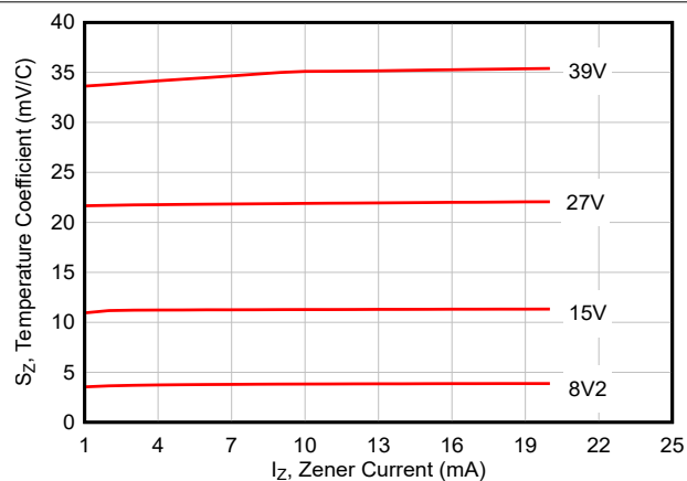
图 5-2. 温度系数
