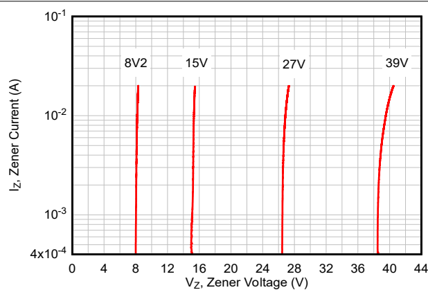
图 5-1. 齐纳电流与齐纳电压间的关系
