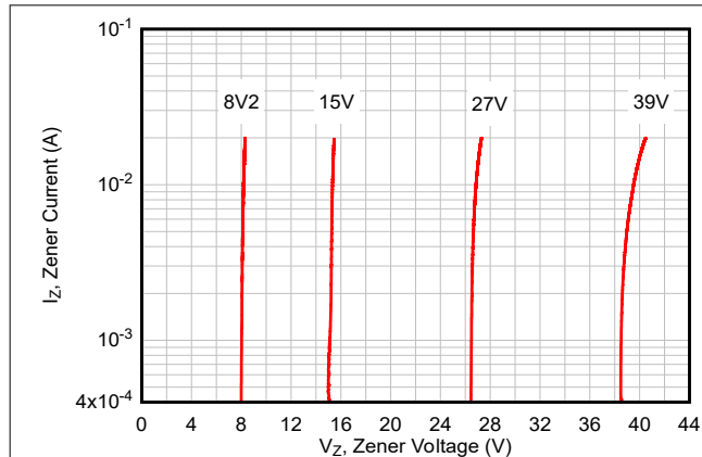
图 5-1. 齐纳电流与齐纳电压间的关系
