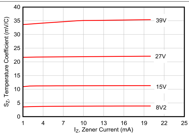
图 5-2. 温度系数
