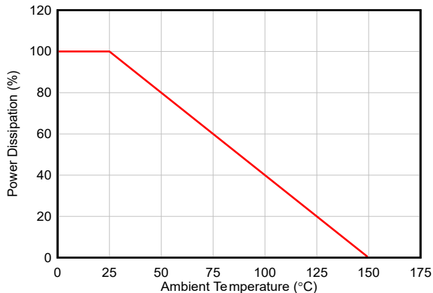
图 5-3. 功率降额曲线
