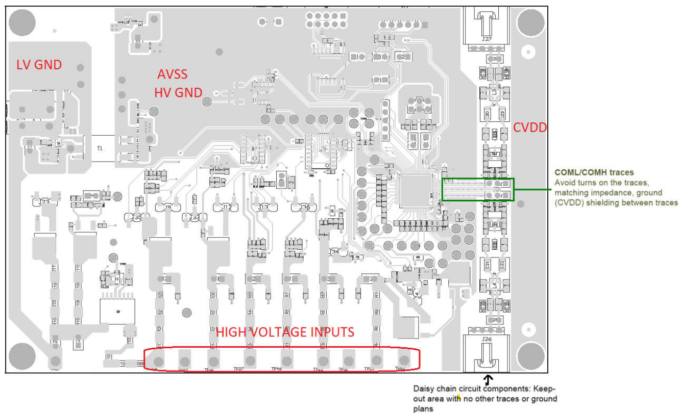
图 11-3. Top Signal Layer
