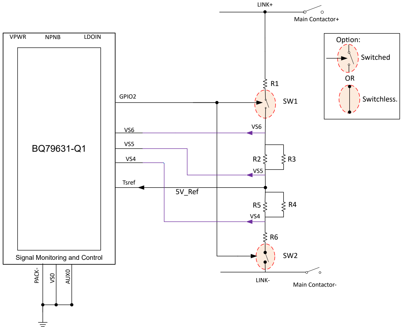
图 9-4. LINK+/- Measurement
