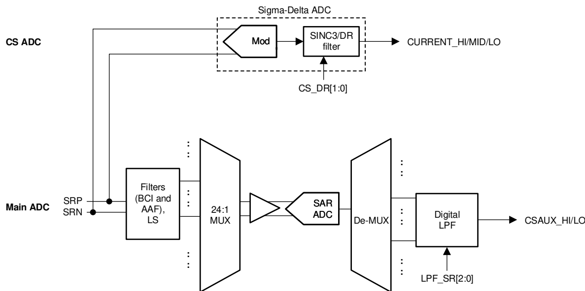
图 8-10. CS ADC
