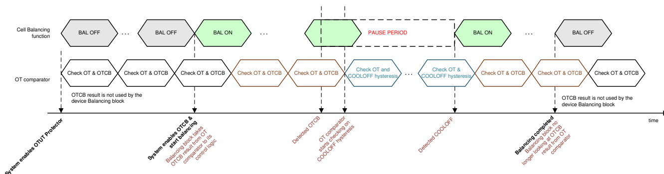
图 8-17. 通过 OTCB 检测暂停和恢复电芯均衡
