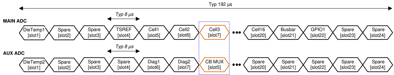
图 8-12. 主 ADC 和 AUX ADC 采样之间的同步
