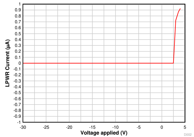
图 8-2. LPWR Current
