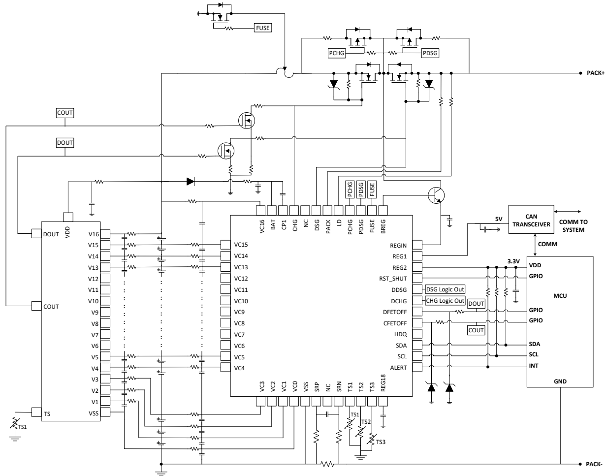
图 8-4. BQ77216 with BQ76952
