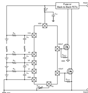
图 3-1. 简化版原理图
