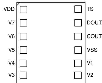
图 5-1. BQ77207 引脚图
