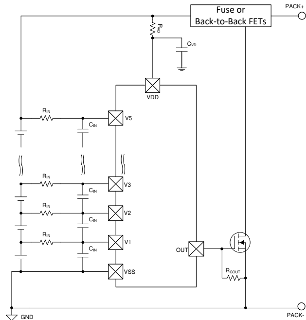
简化原理图
