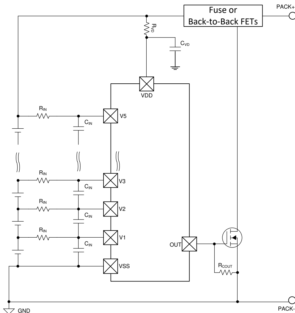
图 8-1. 应用配置
