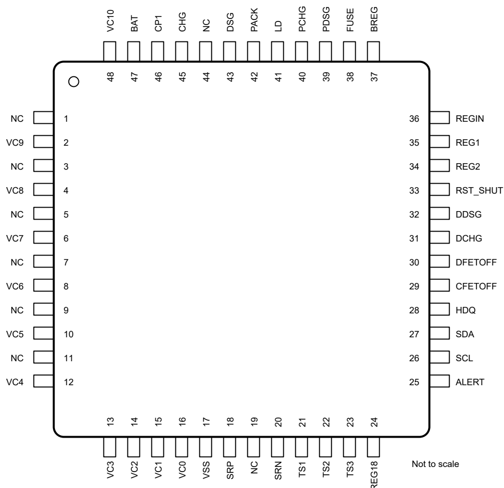
图 6-1. Pinout (top)
