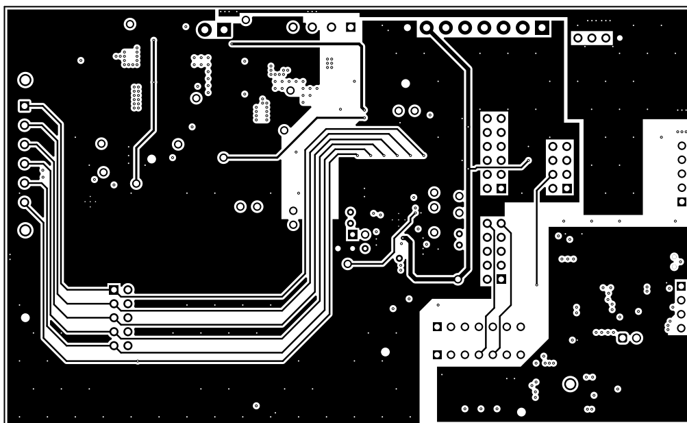
图 10-5. BQ76922EVM Layer 3
