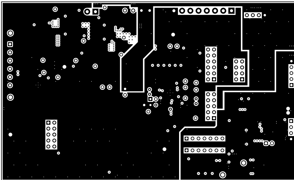
图 10-4. BQ76922EVM Layer 2
