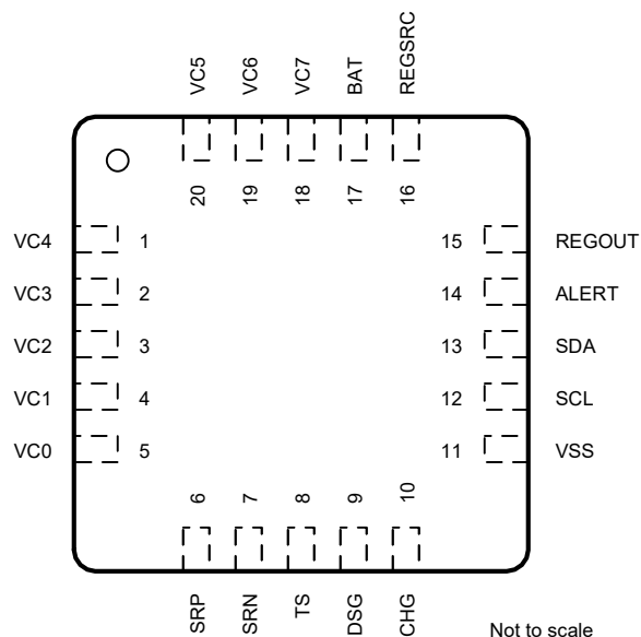
图 5-1. BQ76907-Q1 引脚排列
