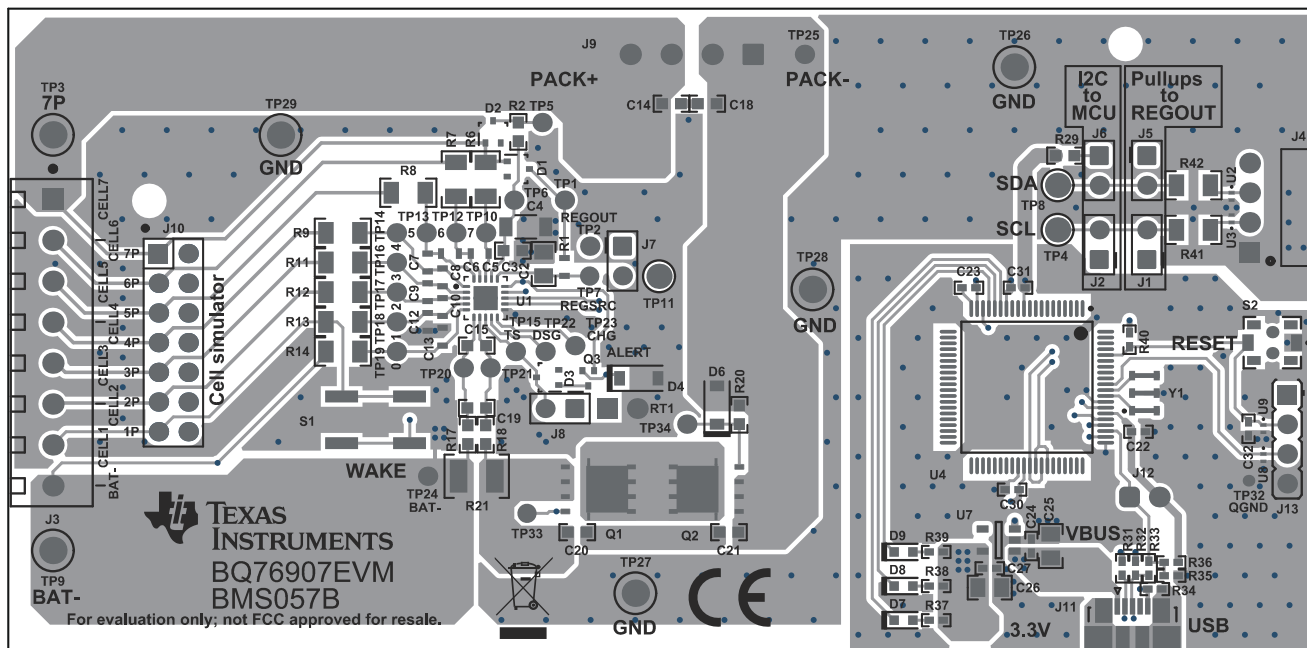
图 8-9. BQ76907-Q1 两层电路板布局布线 - 顶层
