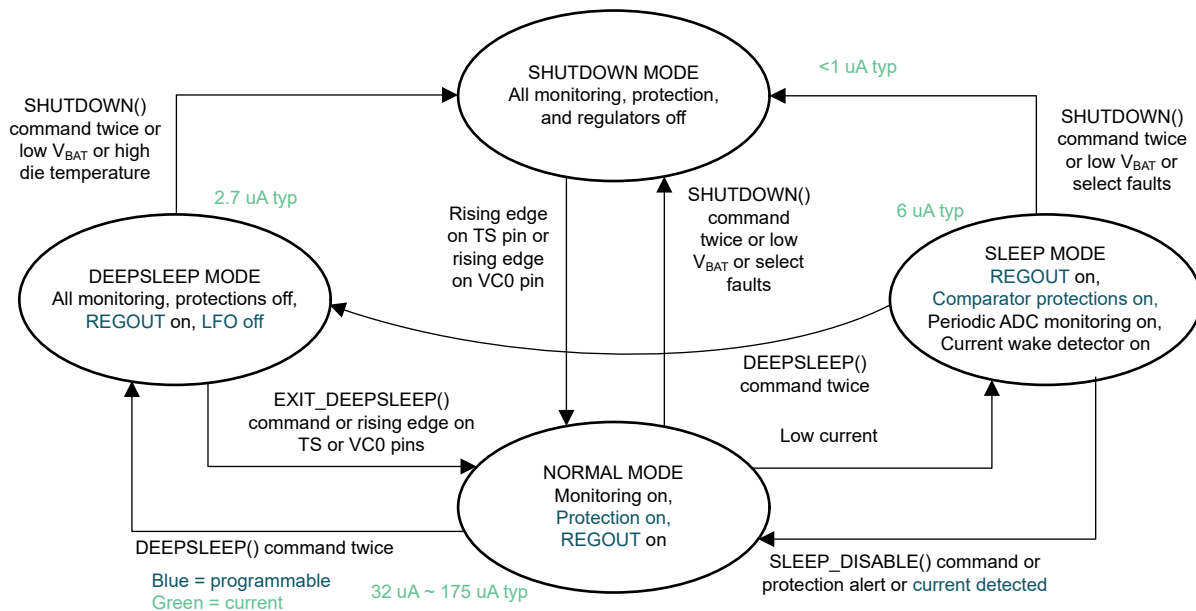
图 7-5. BQ76907-Q1 运行功率模式
