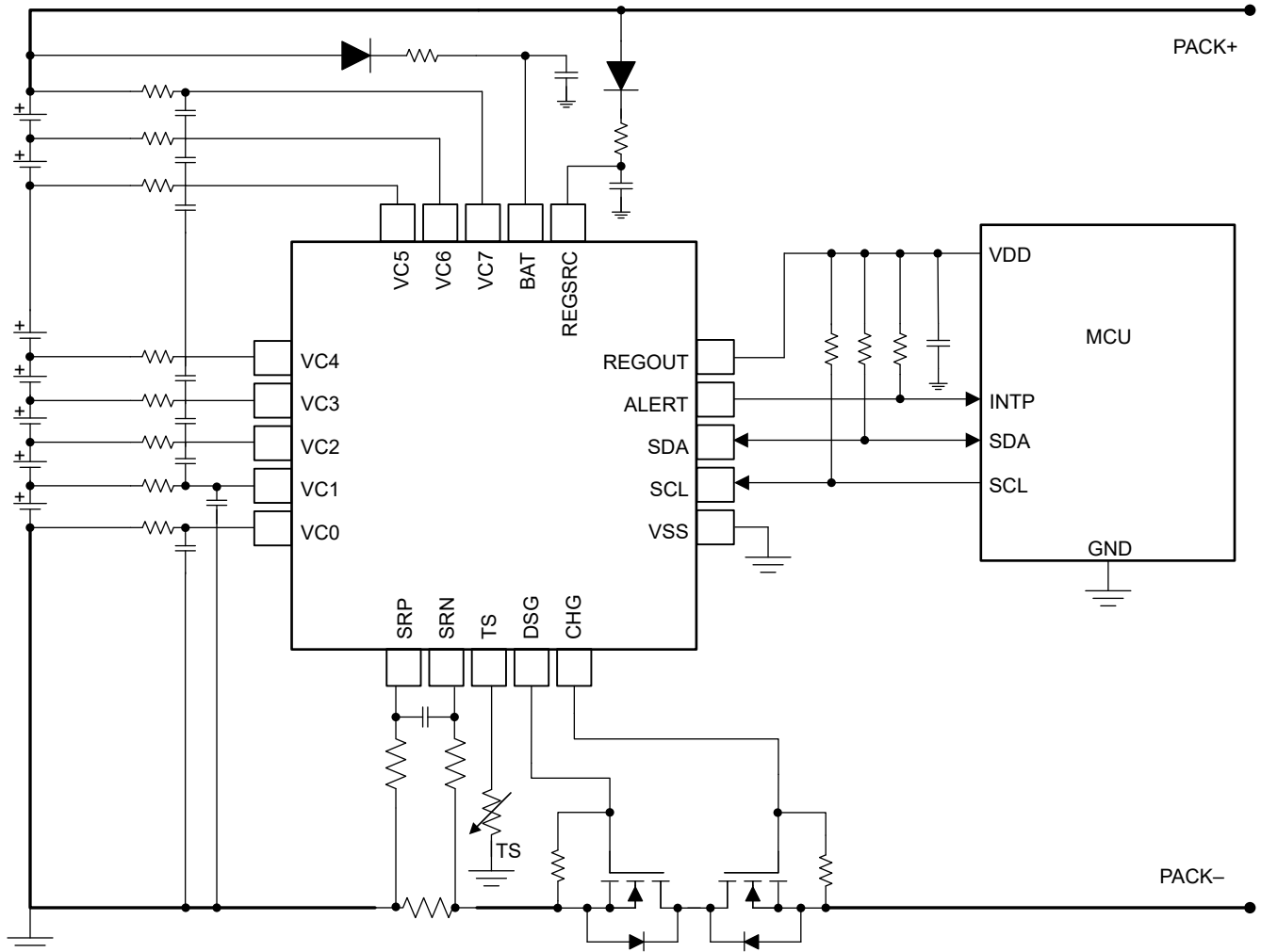
图 8-1. BQ76907-Q1 7 节串联电芯典型实现方式 ( 简化原理图 )
