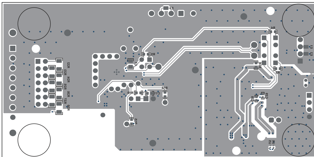
图 8-10. BQ76907-Q1 两层电路板布局布线 - 底层
