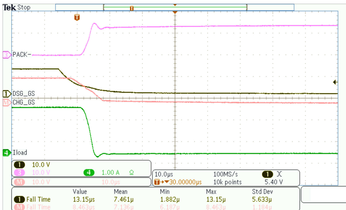
图 8-6. 中速 FET 关断，使用一个 1.35\text{k}\Omega 串联栅极电阻，并且 PACK+ 和 PACK- 之间具有 2A 负载。
