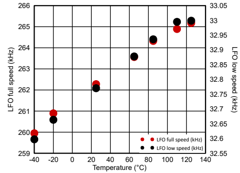
图 6-19. 低频振荡器 (LFO) 精度与温度间的关系
