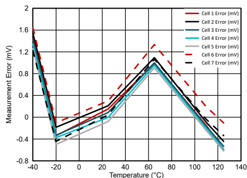
图 6-10. 电芯电压为 4.0V 时电芯电压测量误差与温度间的关系
