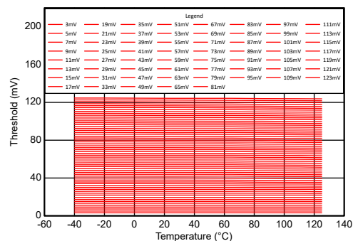
图 6-21. 充电过流保护 (OCC) 阈值与温度间的关系
