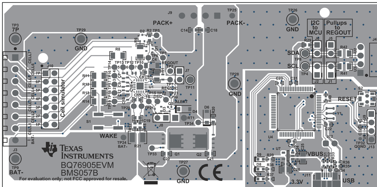
图 8-9. BQ76905 两层电路板布局布线 - 顶层
