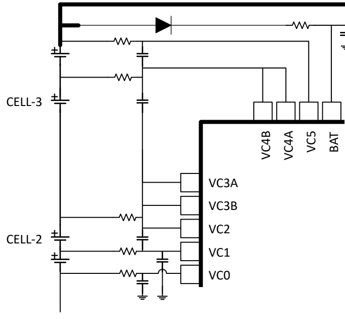
图 7-5. 连接未使用的电芯输入引脚
