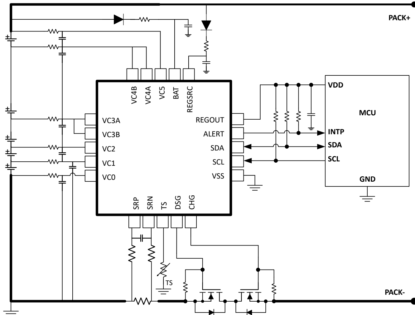
图 8-1. BQ76905 5 节串联电芯典型实现方式 ( 简化原理图 )
