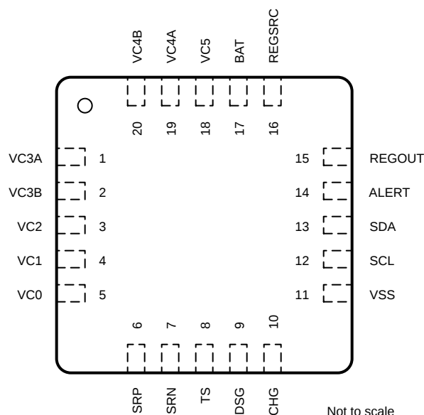
图 5-1. BQ76905 引脚排列
