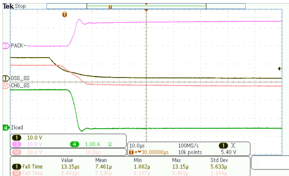
图 8-6. 中速 DSG FET 关断，使用一个 1.35\text{k}\Omega 串联栅极电阻，并且 PACK+ 和 PACK- 之间具有 2A 负载。
