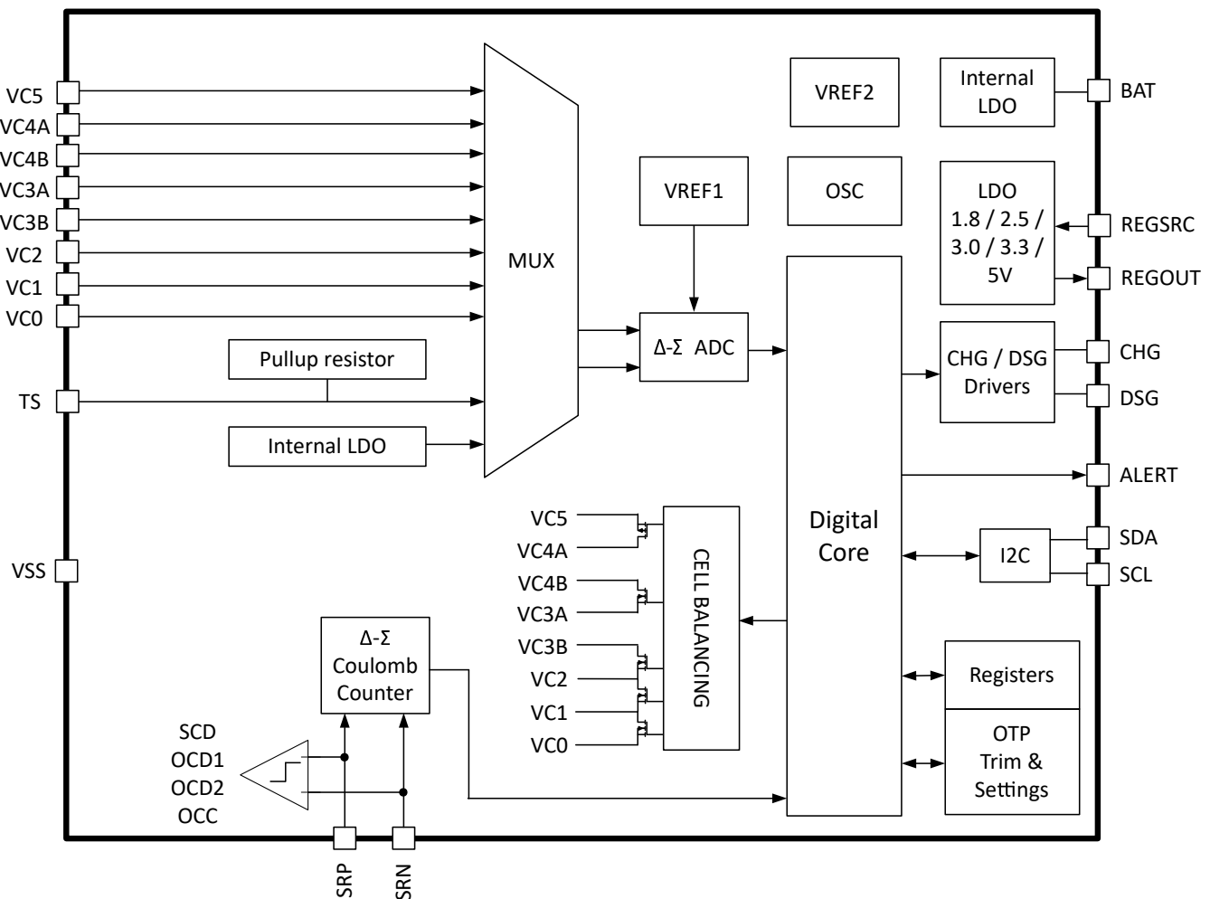
图 7-1. BQ76905 方框图
