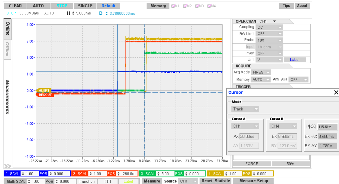
图 8-5. 5 节串联电池包的启动序列
