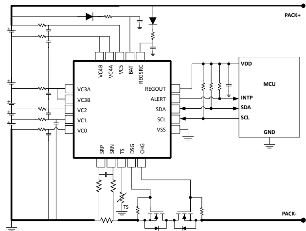
图 3-1. 简化原理图
