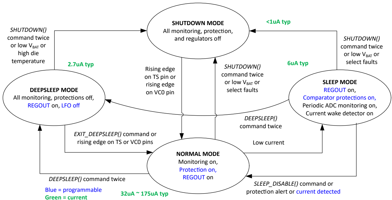
图 7-6. BQ76905 运行功率模式
