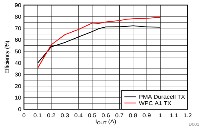
双路模式效率 (5V 输出)
