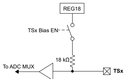
图 4-12. TSx 引脚
