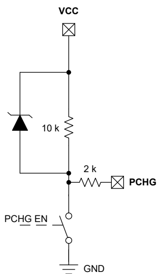
图 4-10. PCHG 引脚
