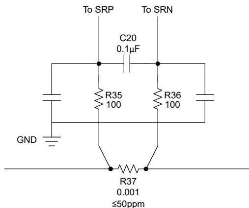
图 7-6. 差分滤波器
