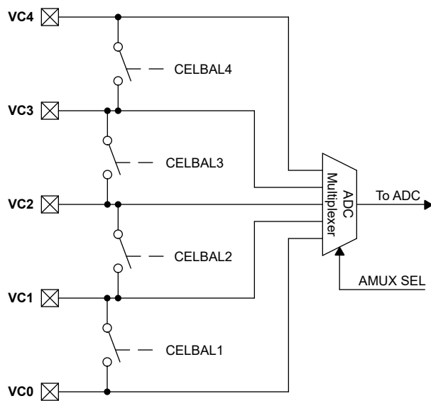
图 4-3. VCx 引脚
