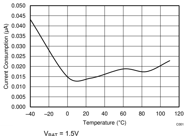
图 6-1. 1.5V I_{BAT} Versus Temperature
