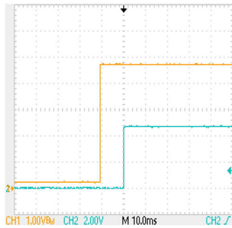
图 9-2. UVP Recovery
