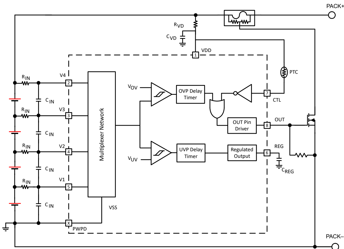
图 7-1. BQ2969T 方框图
