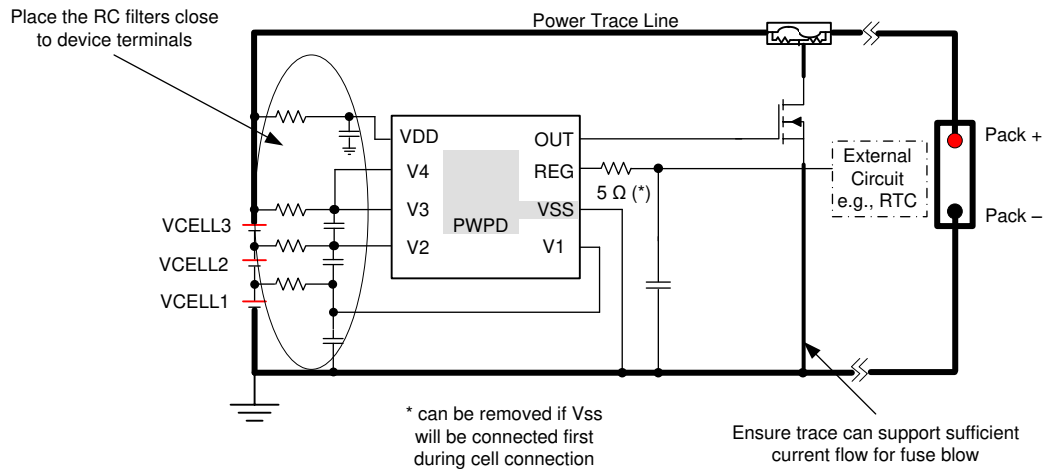
图 10-1. 布局示例
