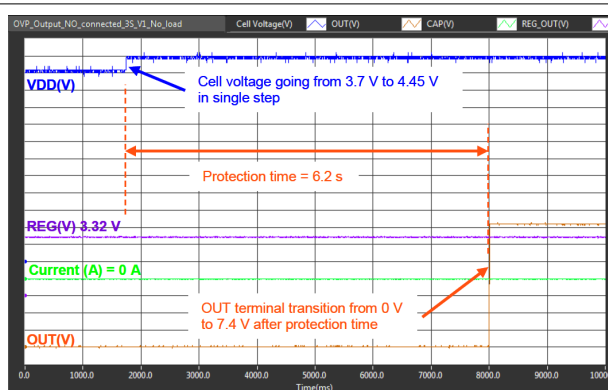
图 8-4. 过压保护
