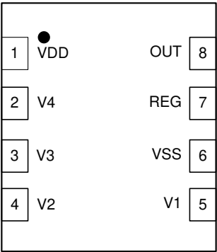
图 5-1. 2 节至 4 节串联电池组 BQ2961 ( 顶视图 )
