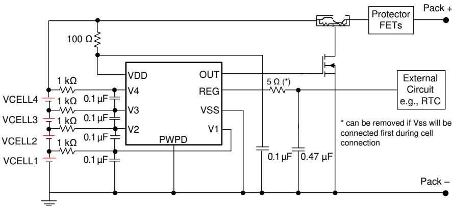
图 8-1. 应用原理图
