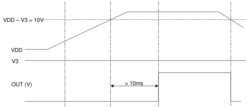
图 7-3. 客户测试模式的时序
