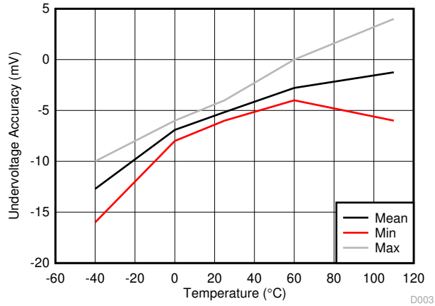
图 6-3. 欠压精度
