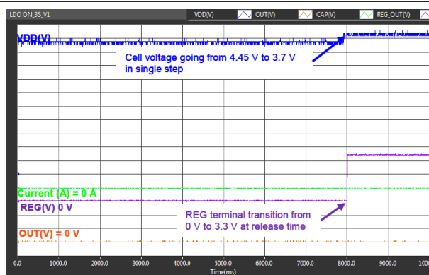
图 8-7. 欠压释放并打开稳压器
