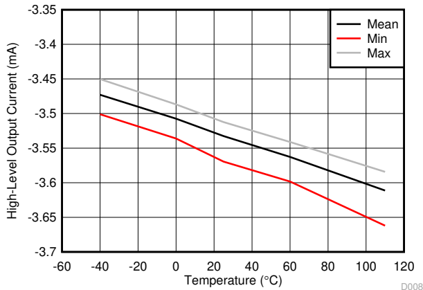
图 6-7. I_{OUTH} 与温度间的关系
