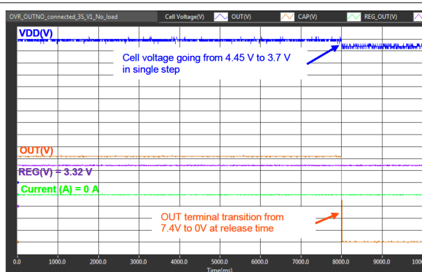
图 8-5. 过压保护释放
