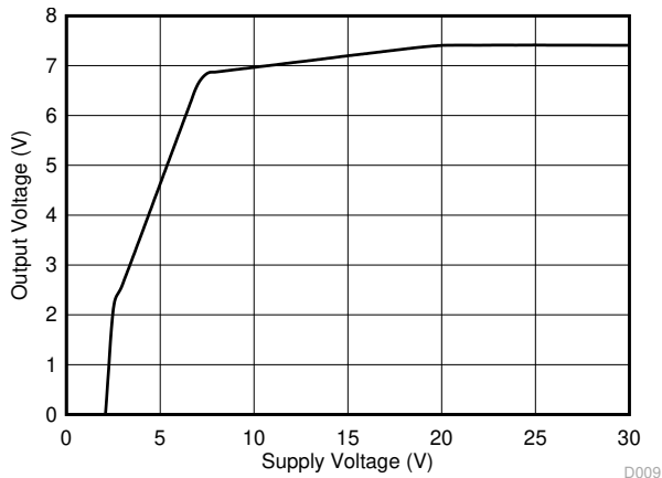
图 6-8. V_{OUT} 与 V_{DD} 间的关系
