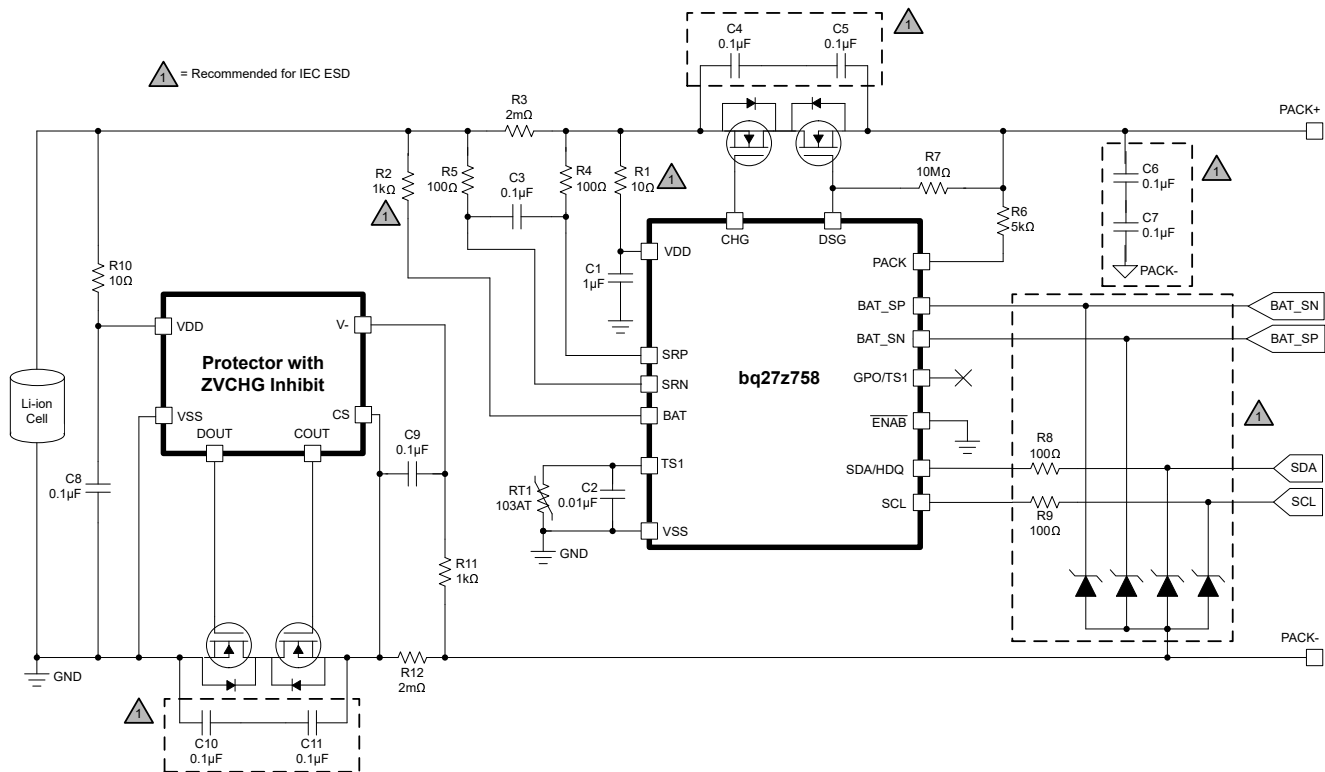
图 7-1. BQ27Z758 具有额外保护器的 1 节串联电芯高侧电流检测典型实现方式 (推荐)
