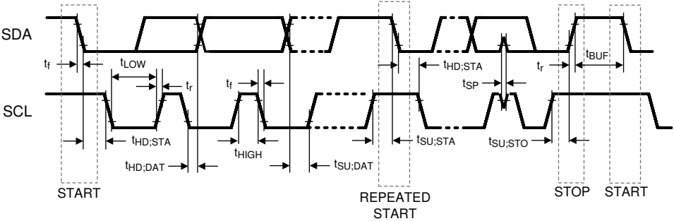
图 5-1. I 2 C 时序
