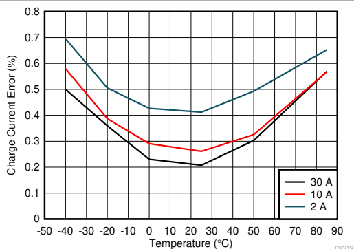
图 5-3. 使用 1\text{m}\Omega 检测电阻时充电电流误差与温度和充电器电流间的关系，无校准
