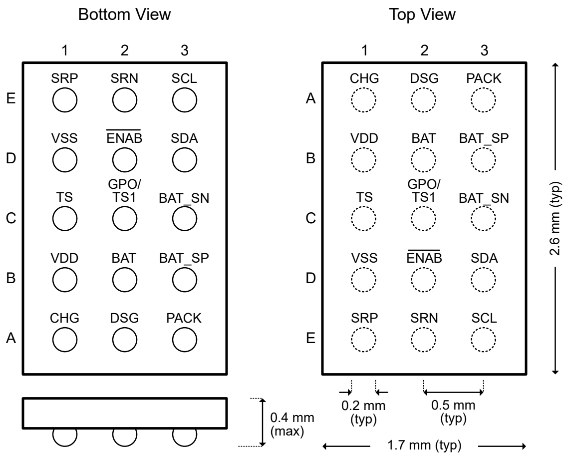
图 4-1. 引脚排列图
