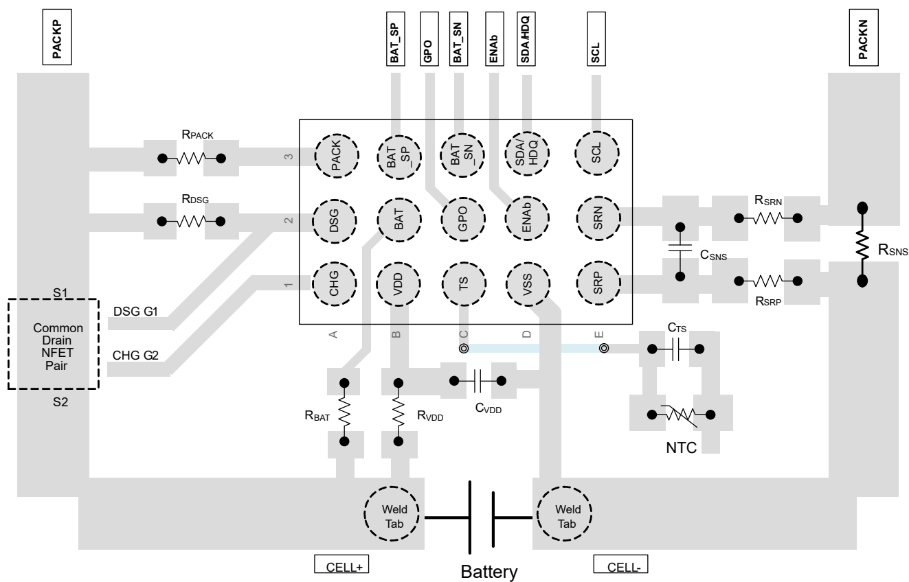
图 9-1. BQ27Z746 主要布线电路板布局布线
