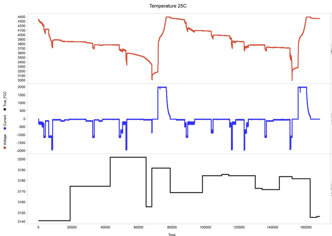
图 7-3. 充满电容量跟踪 (X 轴为秒)
