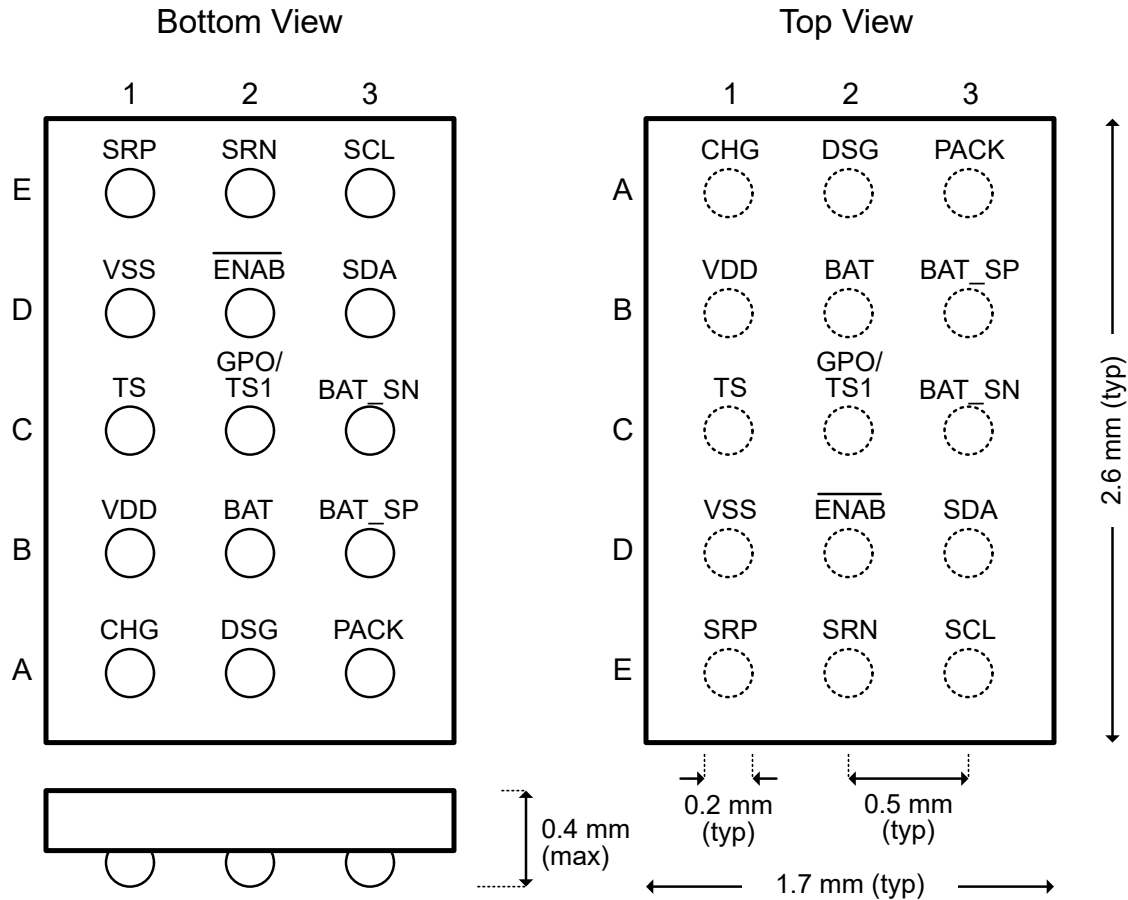
图 4-1. 引脚排列图
