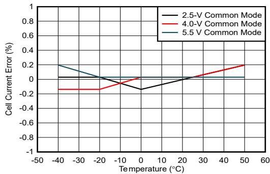
图 5-5. 2.2A 电流误差与 CC ADC 输入共模电压和温度间的关系，无校准
