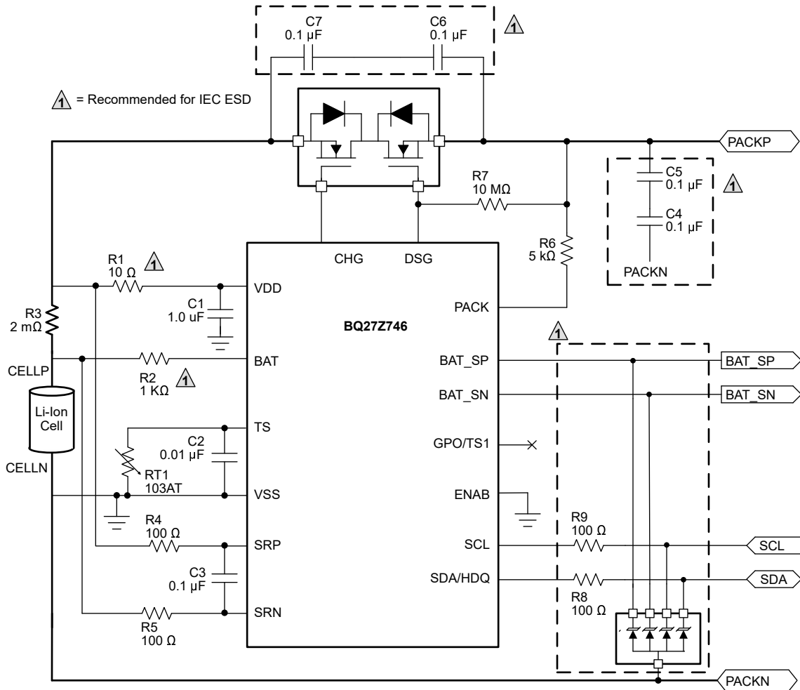
图 7-2. BQ27Z746 1 节串联电芯高侧电流检测典型实现方式
