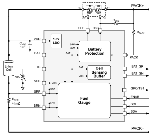
BQ27Z746 简化原理图
