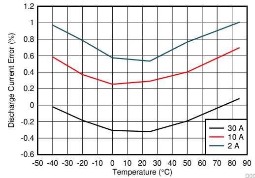
图 5-4. 使用 1\text{m}\Omega 检测电阻时放电电流误差与温度和负载电流间的关系，无校准
