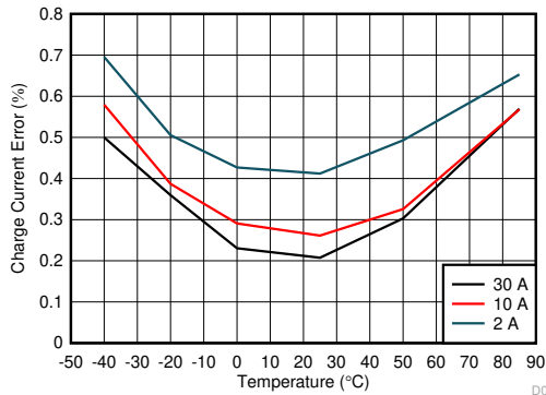
图 5-3. 使用 1\text{m}\Omega 检测电阻时充电电流误差与温度和充电器电流间的关系，无校准
