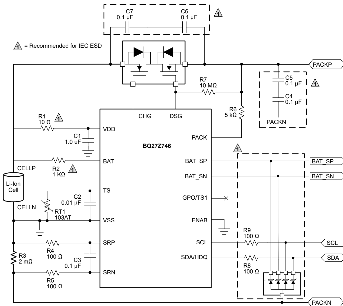
图 7-1. BQ27Z746 1 节串联电芯低侧电流检测典型实现方式
