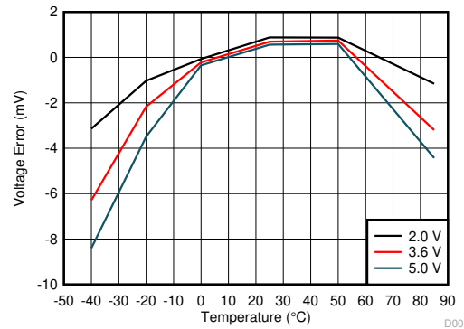
图 5-6. 电芯电压误差与电池电压和温度间的关系
