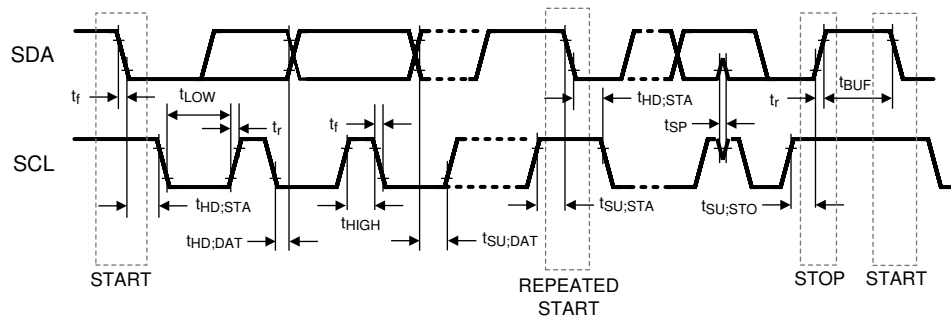
图 7-1. I²C Timing
