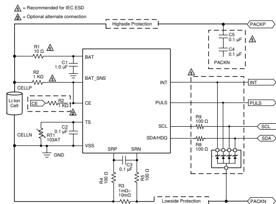
简化原理图
