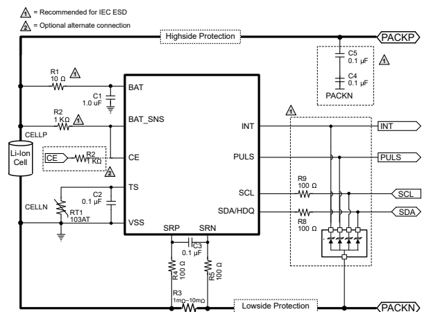
简化原理图
