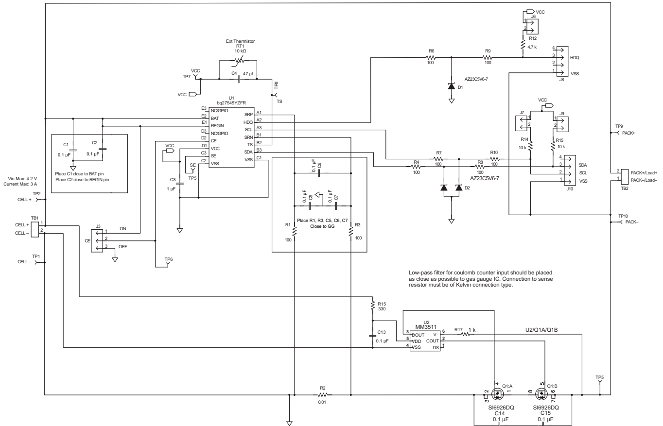
图 9. Reference Schematic
