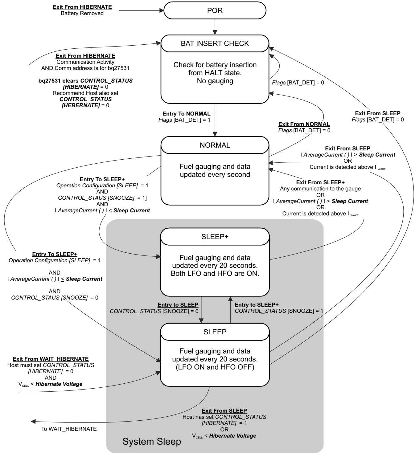
图 8-1. Power Mode Diagram—System Sleep
