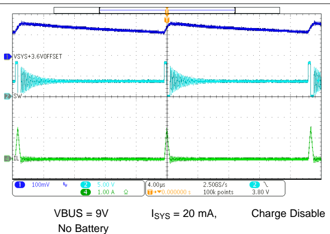
图 46. PFM Switching Waveform
