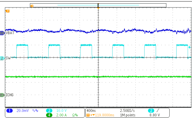
图 48. Charge Enable
