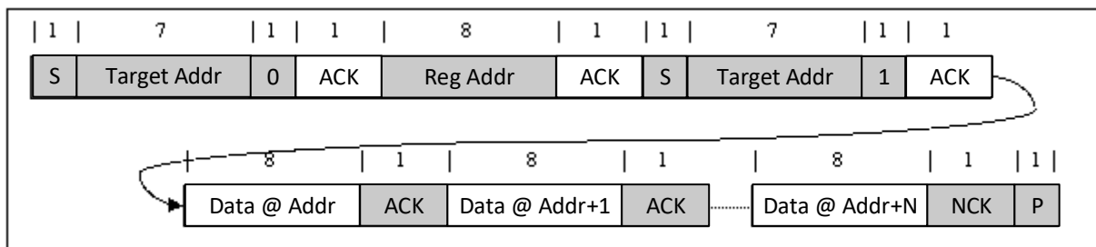
图 8-16. Multi-Read
