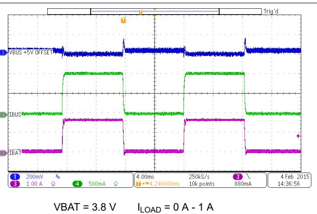
图 9-13. Boost Mode Load Transient
