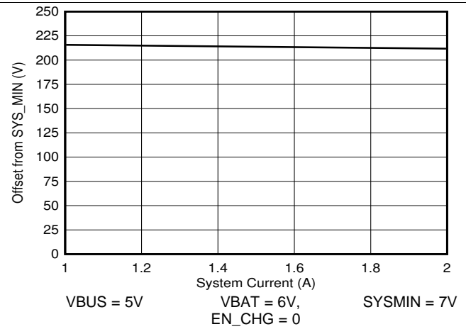
图 8. SYSMIN Load Regulation
