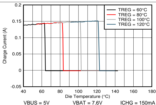
图 16. TREG Profiles
