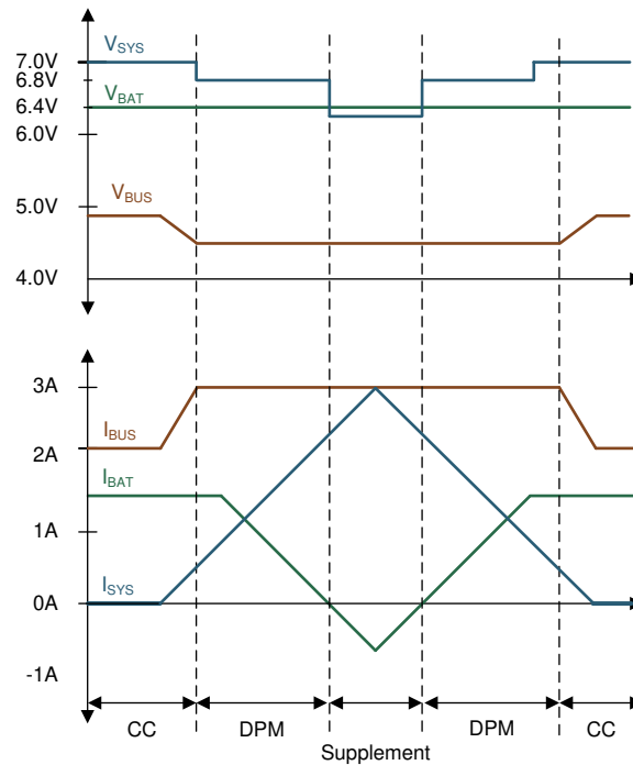
图 20. DPM Response
