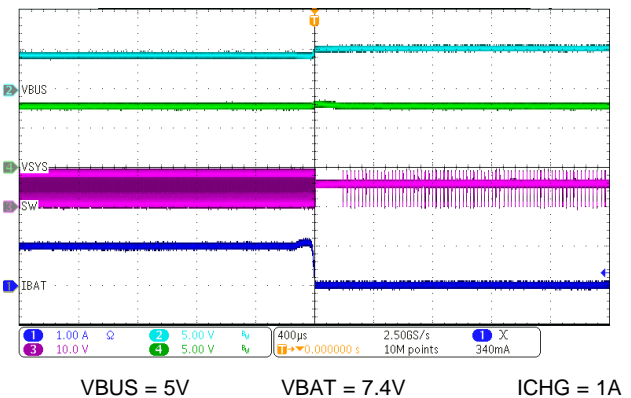
图 79. Charge Disable
