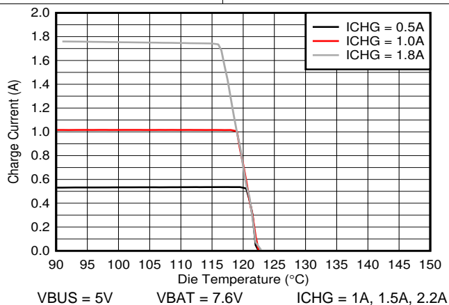
图 17. Max Current Temperature Profile
