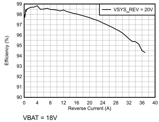
图 5-10. 反向模式效率 (高达 40A)
