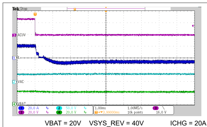
图 7-9. 在 VAC = 30V 及 5A SYS 负载下，从正向模式快速传输到反向模式
