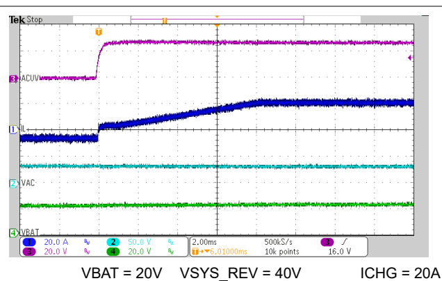
图 7-10. 在 VAC = 30V 及 5A SYS 负载下，从反向模式快速传输到正向模式
