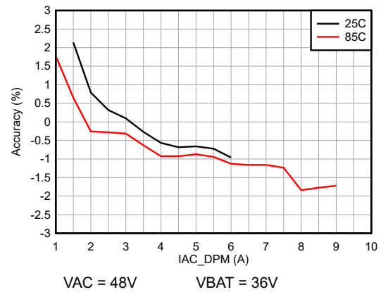
图 5-8. 输入电流 (IAC_DPM) 调节精度 (在不同的温度下)
