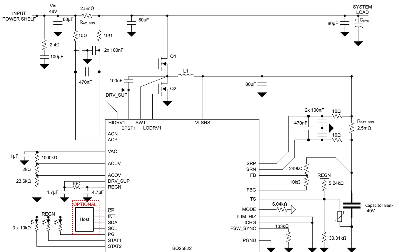
图 7-1. BQ25822：高功率超级电容器备用应用示意图
