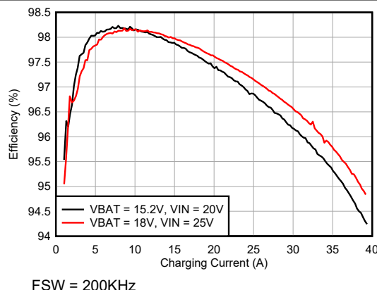
图 5-4. 充电效率与充电电流间的关系 (高达 40A)
