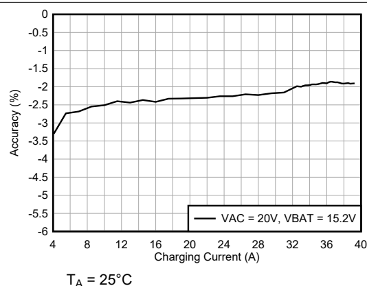
图 5-6. 充电电流精度 (高达 40A)
