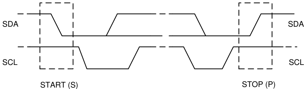
图 6-8. I 2 C 总线上的 START 和 STOP 条件
