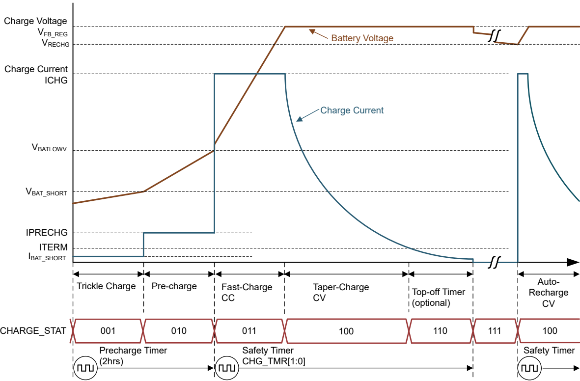
图 6-3. 典型的锂离子电池充电曲线
