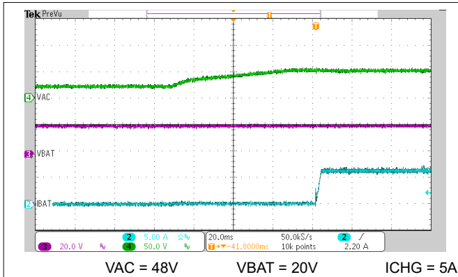
图 7-3. 5A ICHG 下的 VAC 插入上电
