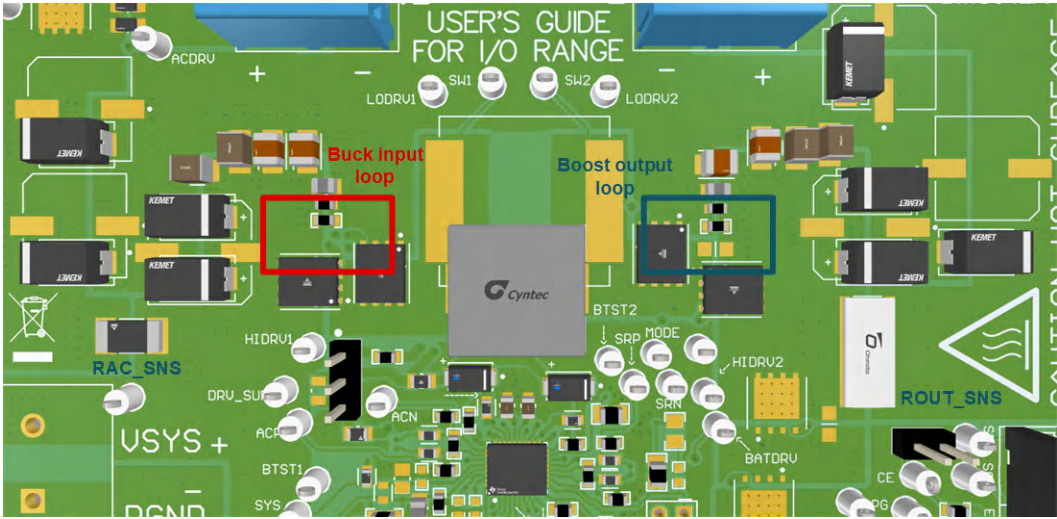
图 7-11. PCB 布局参考示例顶视图
