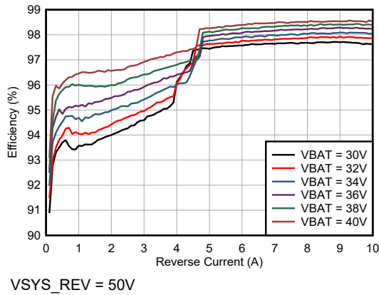
图 5-9. 反向模式效率
