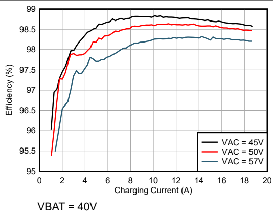
图 5-3. 充电效率与充电电流间的关系
