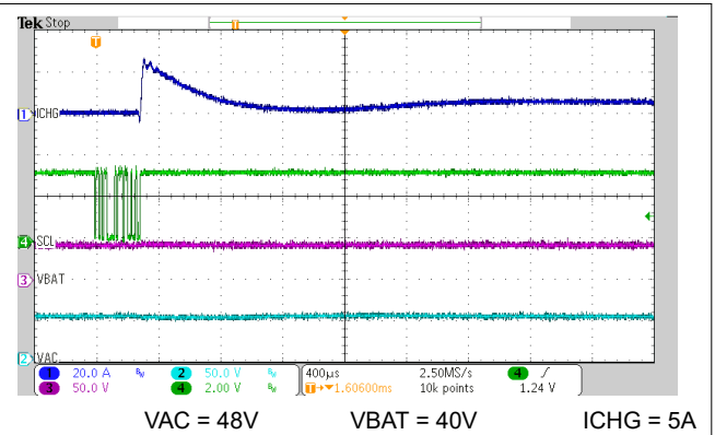
图 7-4. 5A ICHG 下通过 I 2 C 实现的充电启用
