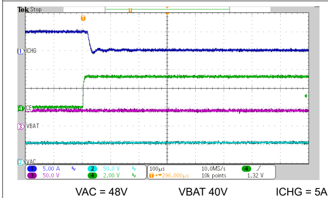
图 7-7. 5A ICHG 下通过 \overline{CE} 引脚实现的充电禁用
