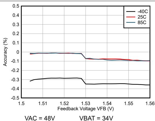
图 5-5. 反馈电压精度 (在不同的温度下)
