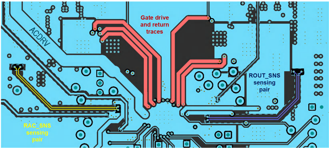
图 7-12. PCB 布局栅极驱动和电流检测信号层布线
