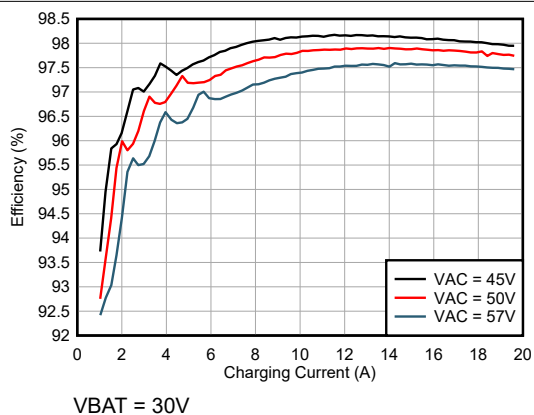
图 5-1. 充电效率与充电电流间的关系
