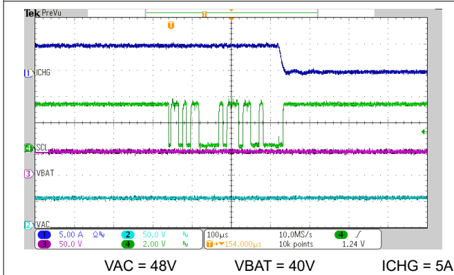
图 7-5. 5A ICHG 下通过 I 2 C 实现的充电禁用
