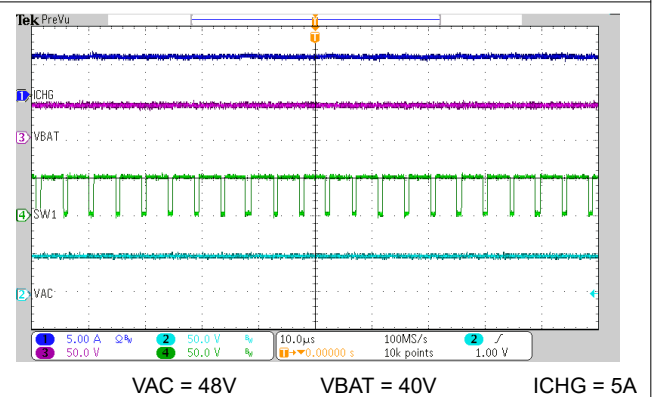
图 7-8. 降压开关波形
