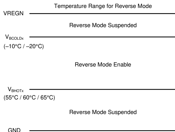
图 6-5. 反向模式下的 TS 引脚热敏电阻检测阈值
