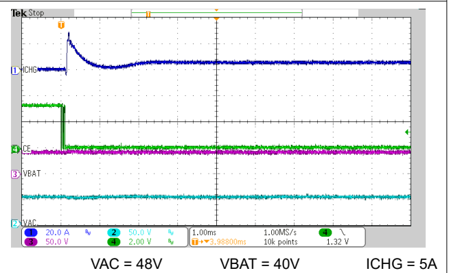
图 7-6. 5A ICHG 下通过 \overline{CE} 引脚实现的充电启用
