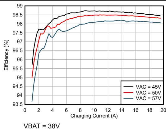
图 5-2. 充电效率与充电电流间的关系
