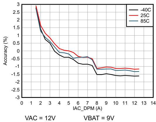
图 5-7. 输入电流 (IAC_DPM) 调节精度 (在不同的温度下)
