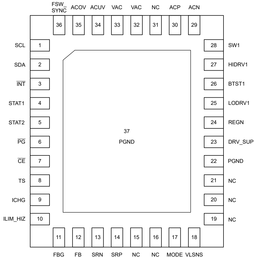
图 4-1. BQ25822 RRV 封装 36 引脚 VQFN 顶视图
