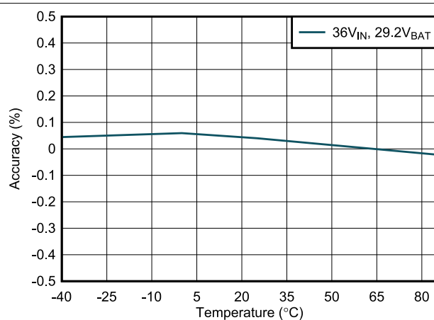
图 6-4. 充电电压精度与温度间的关系
