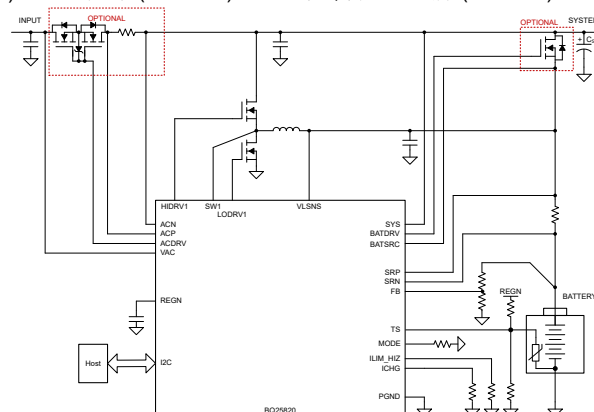
BQ25820 简化原理图
