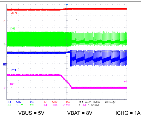
图 10-7. Charge Disable
