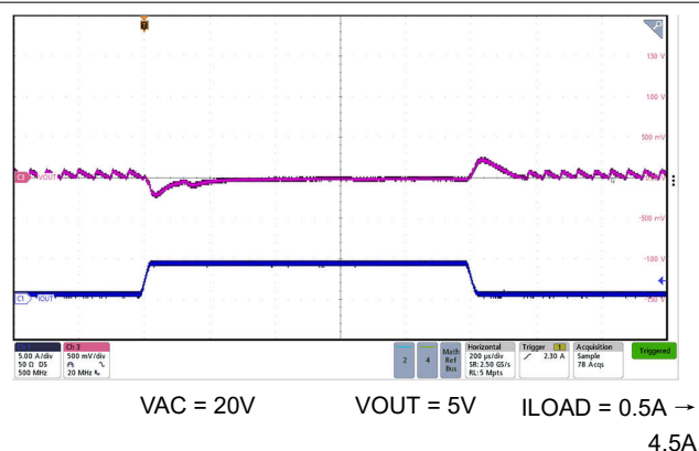
图 7-11. 输入电压为 20V 时的正向模式 5V 瞬态响应
