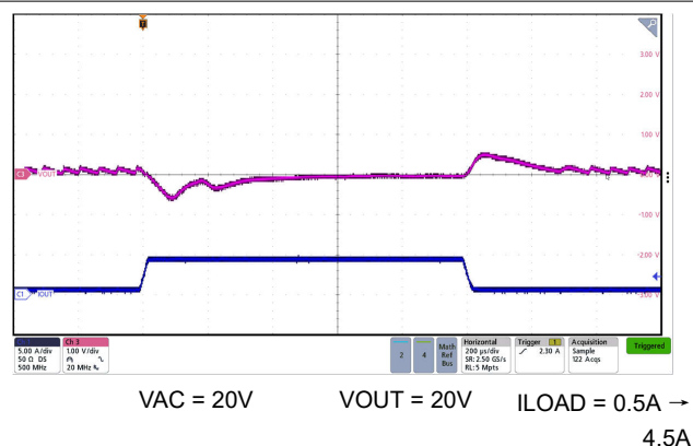
图 7-13. 输入电压为 20V 时的正向模式 20V 瞬态响应
