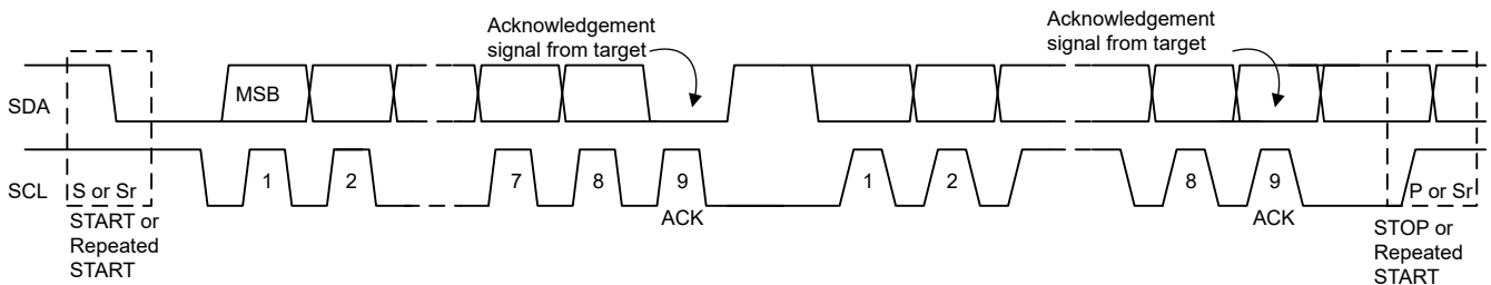
图 6-9. I²C 总线上的数据传输
