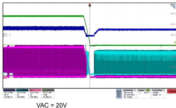
图 7-10. 输出短路响应
