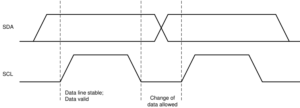
图 6-7. I²C 总线上的位传输
