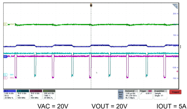
图 7-9. 降压/升压开关波形
