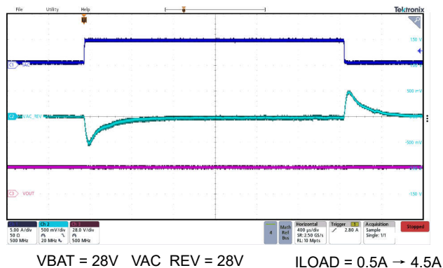
图 9-16. 反向模式降压/升压瞬态响应
