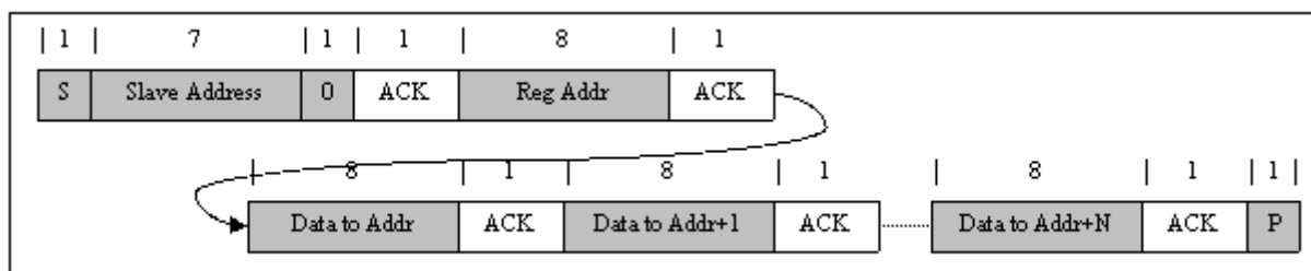
图 9-14. Multi Write
