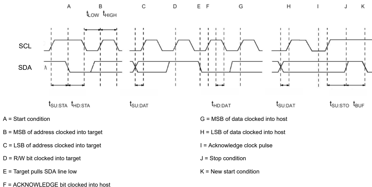
图 9-7. SMBus Read Timing
