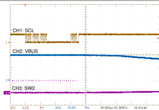
图 10-18. OTG Power Off
