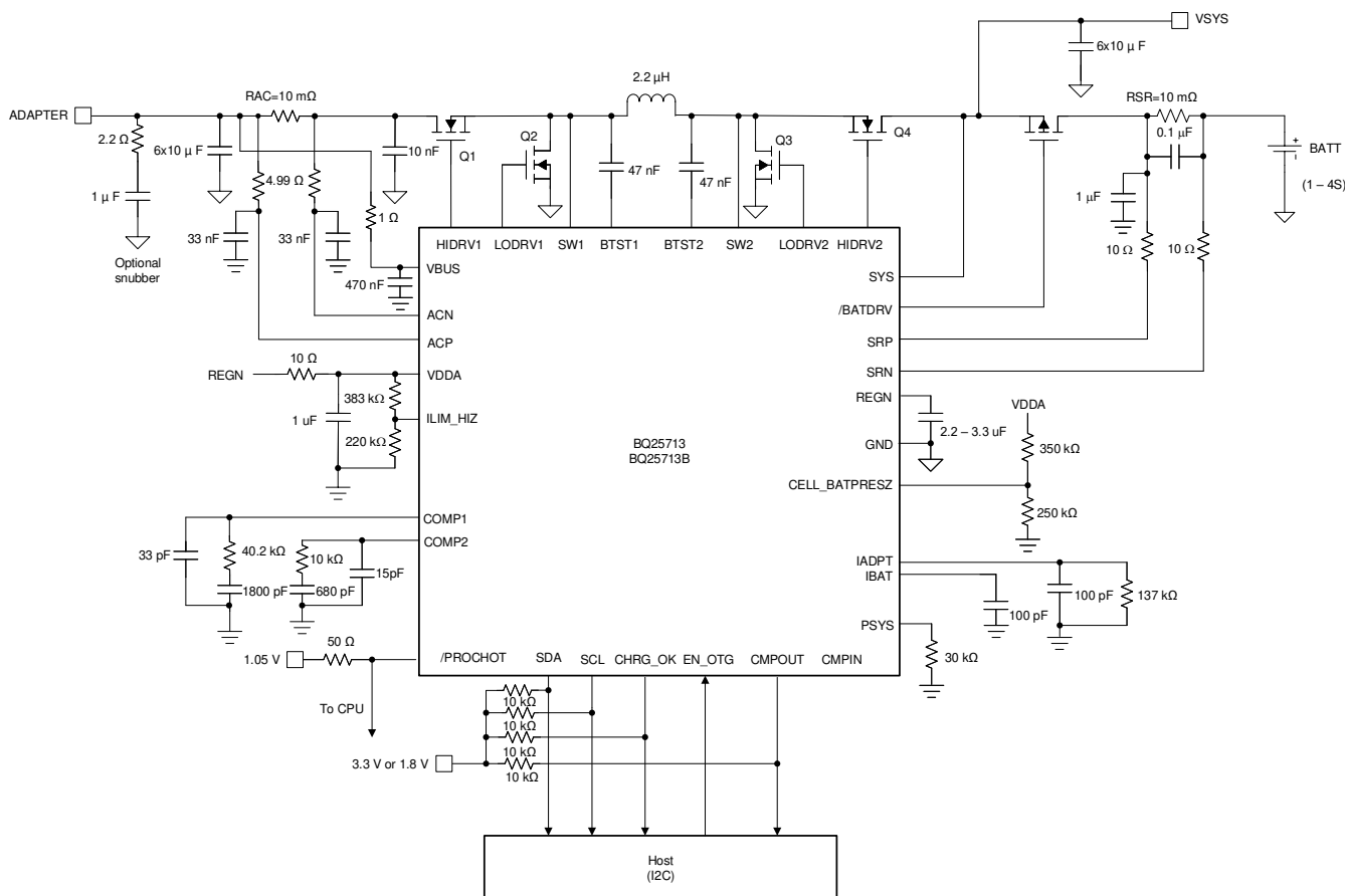
图 10-1. 应用示意图
