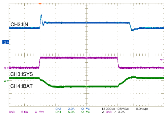
图 10-15. 升压模式下的输入电流
