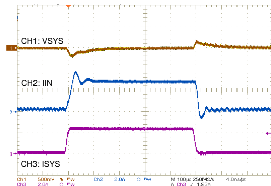
图 10-10. 降压/升压模式期间切换
