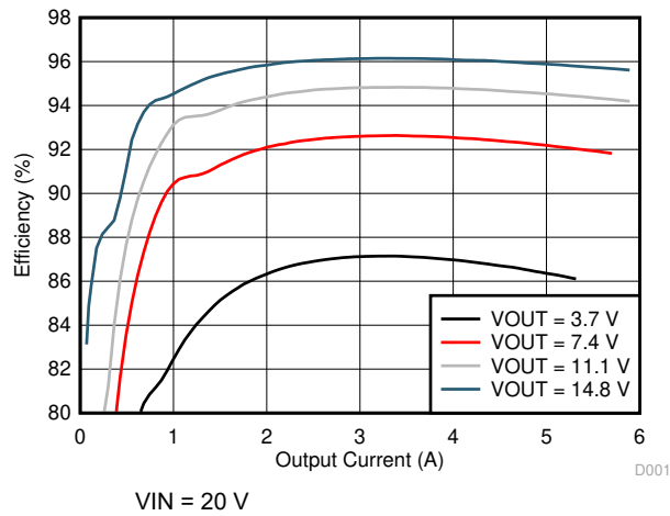
图 8-7. 系统效率
