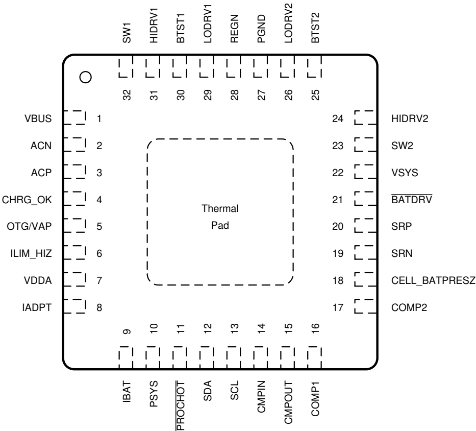
图 7-1. RSN 封装 32 引脚 WQFN 顶视图
