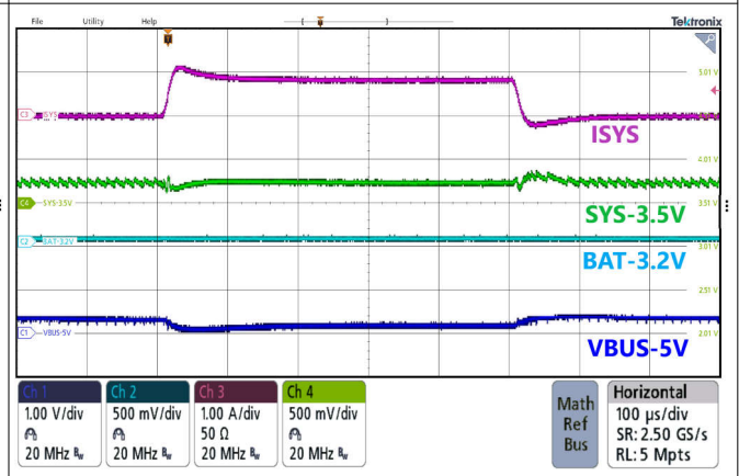
图 8-5. Charge Enable
