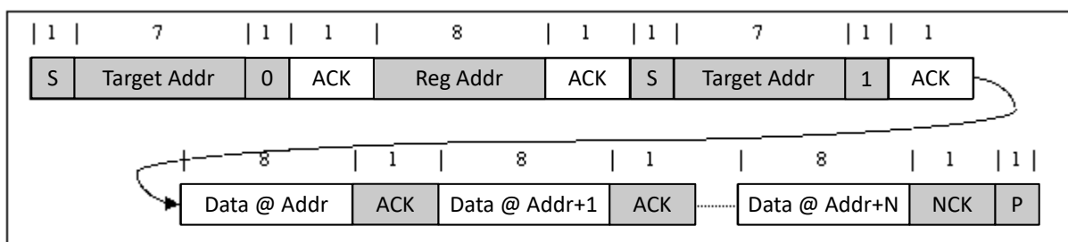
图 8-16. 多重读取
