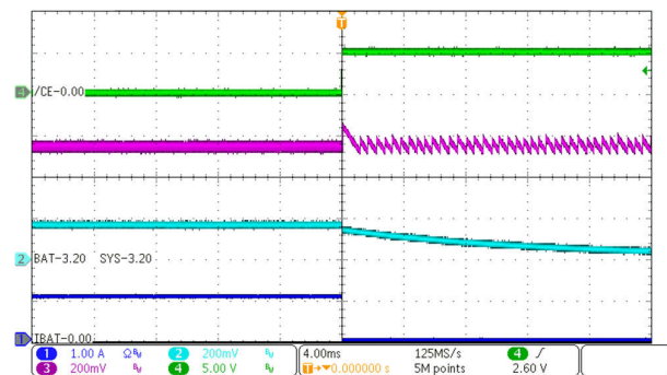
图 9-4. 断电
