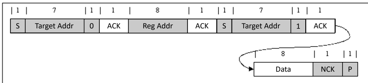
图 8-14. 单次读取
