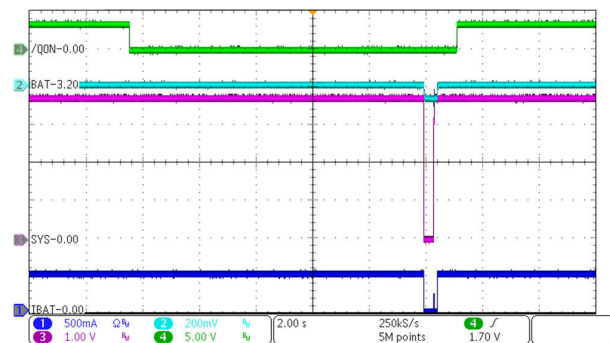
图 9-6. 充电禁用
