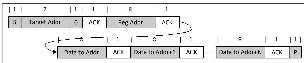
图 8-15. 多重写入
